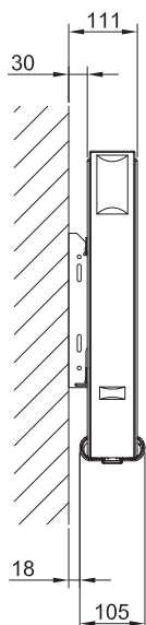
widok z boku
