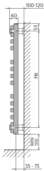
widok z boku
