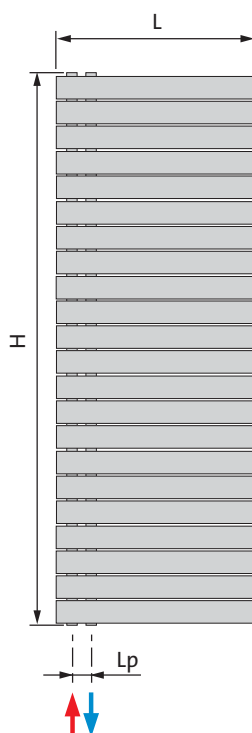
wymiary w mm
