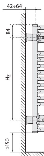
widok z boku
