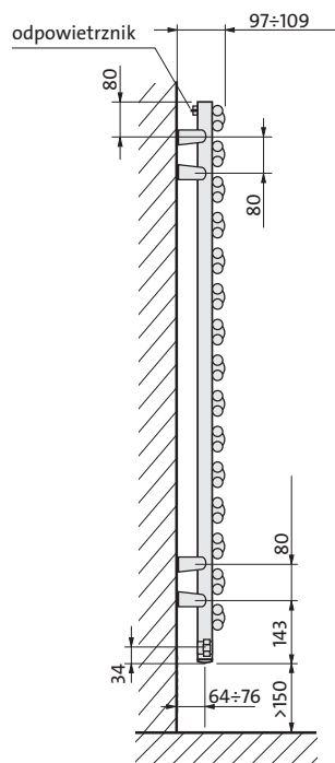
widok z boku
