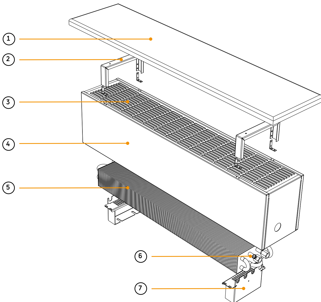
Konstrukcja grzejników Aura Bench WDF
