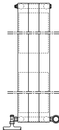
podłączenie dolne z prawej
