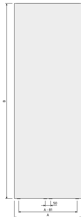
rzuty z boku
