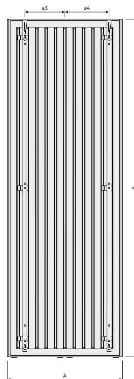
odległości montażowe [mm]
