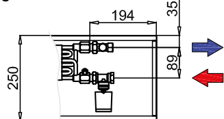
F1S-25 wysokość: 75 mm
