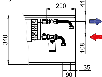
F2C-34 / F2V-34 wysokość: 170 mm
