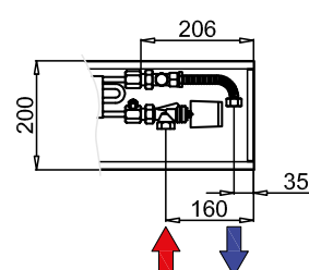
F1S-20 wysokość: 75 mm
