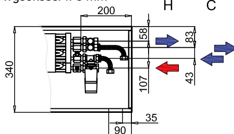
F4C-34 / F4V-34 wysokość: 170 mm
