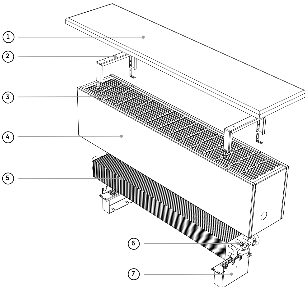
Konstrukcja grzejników Aura Bench
