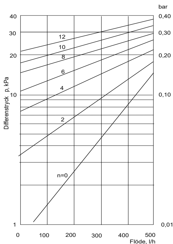
Fjäder för tryckområde 0,2 bar, (0-2 mvp), (0-20 kPa)
