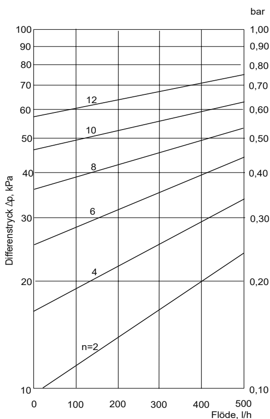
Fjäder för tryckområde 0,1-0,6 bar, (1-6 mvp), (10-60 kPa)
