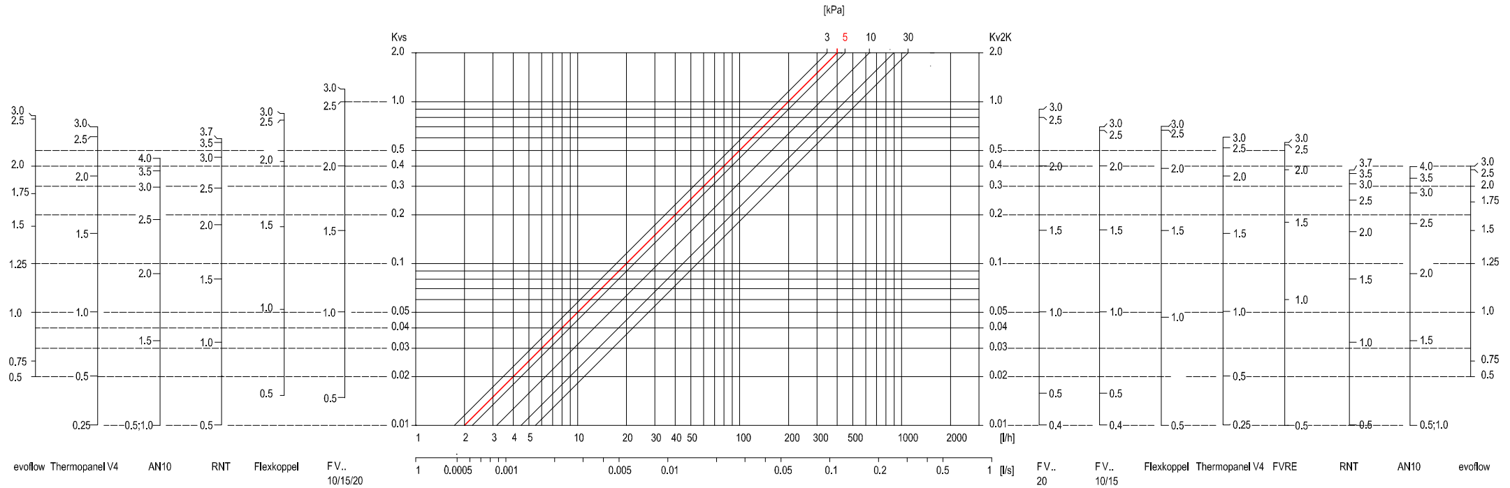
Tryckfallsdiagram
