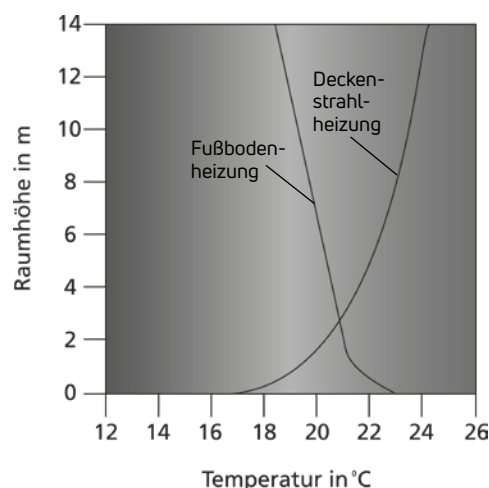
Abb. 87 Temperaturprofil
