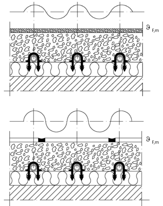
Abb. 134 Temperaturen in der Fußbodenheizung
