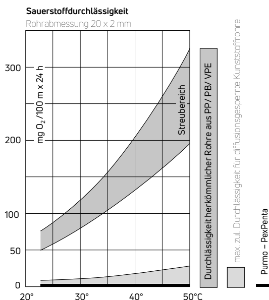
Abb. 1 Sauerstoffdurchlässigkeit Purmo-Heizrohr
