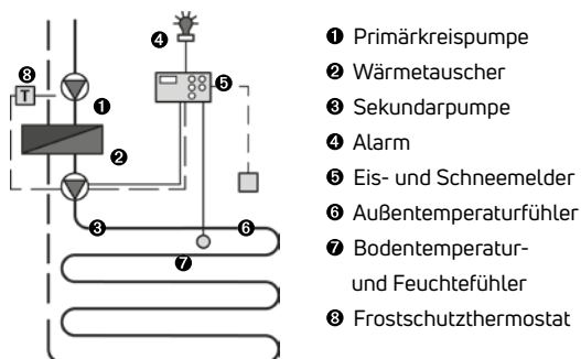
Abb. 90 Schaltschema
