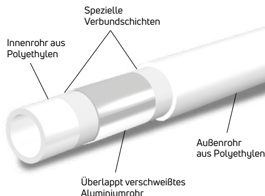
Abb. 6 Aufbau SKR-Heizrohr
