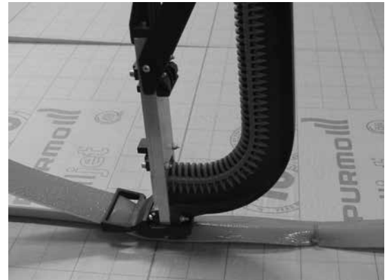
Abb. 138 Bei rolljet Dämmungen lassen sich mit Hilfe der isojet-Dämmung Leitungen schnell und einfach isolieren
