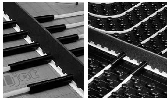
Abb. 131 Dehnfugenprofil rolljet (links) sowie Dehnungsfugenprofil und Übergangselement noppjet uni (rechts)
