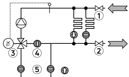
Abb. 114 Füllen und Spülen der einzelnen Heizkreise
