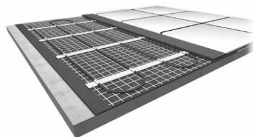
Abb. 92 Bodenbau mit eljet
