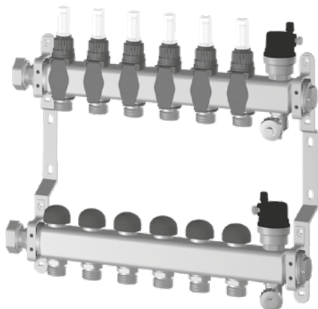
Abb. 99 Heizkreisverteiler Premium line
