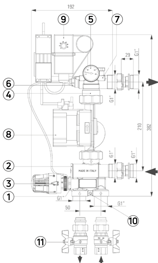
Abb. 112 Prinzipskizze Festwertregelset TempCo fix eco 3
