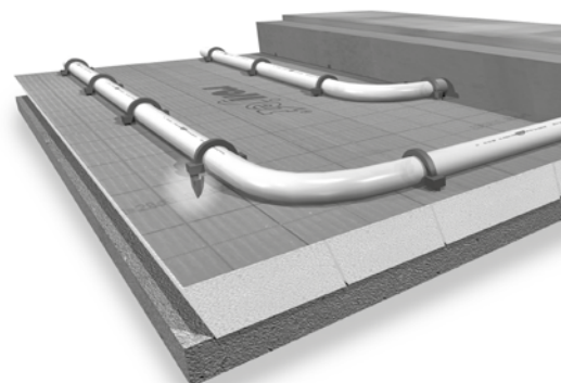
Abb. 15 rolljet
