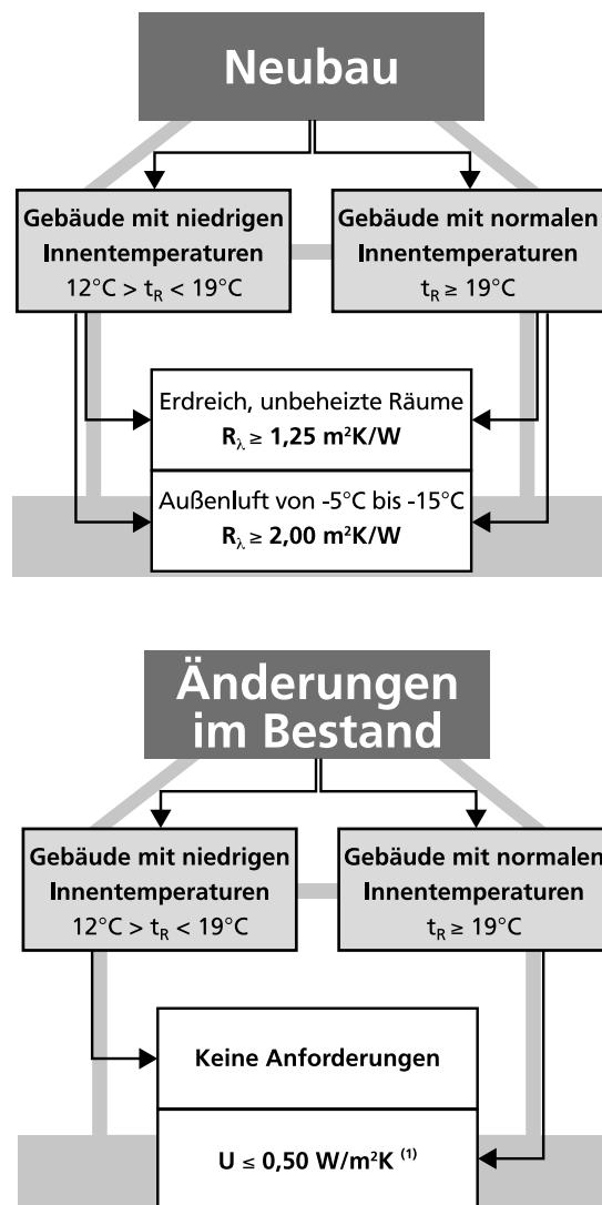
Abb. 129 Anforderungen an Wohnungstrenndecken nach dem GEG
