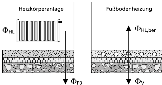
Abb. 135 Wärmeströme durch den Fußboden
