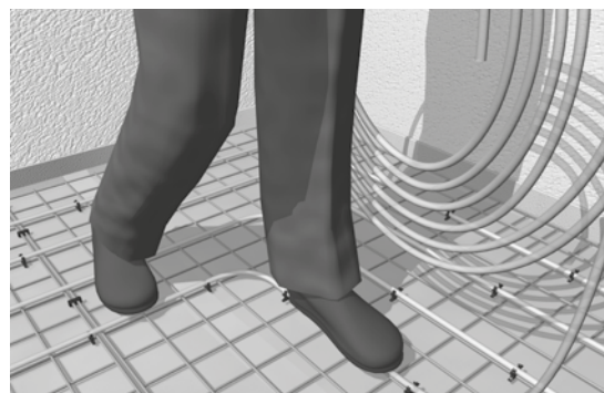
Abb. 59 clickjet Verlegung
