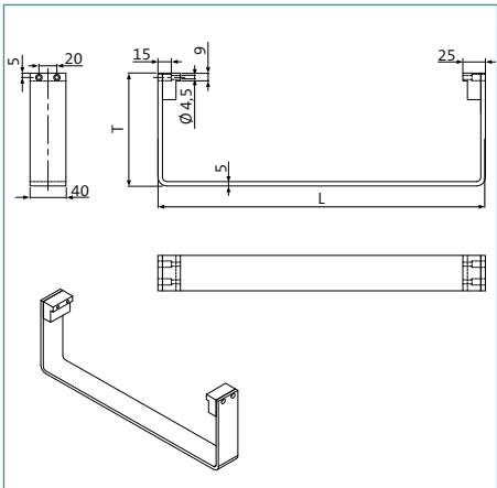
Handtuchstange für Paros V – nimmt perfekt die Linien der sanft gebogenen Seitenabschlüsse auf.
