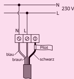
Abb. 110 Elektrischer Anschluss
