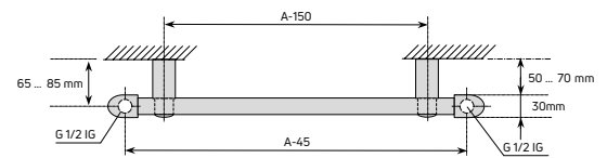
Abb. 67 Anschlussabstände Flores
