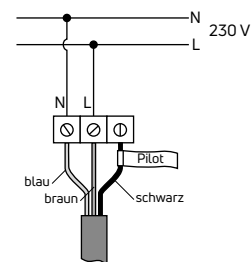
Abb. 98 Elektrischer Anschluss
