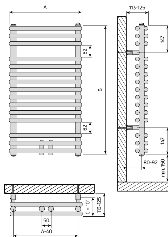
Abb. 83 Abmessungen und Montage Maße
