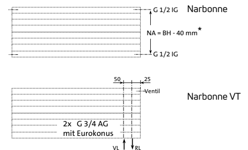
Abb. 64 Anschluss
