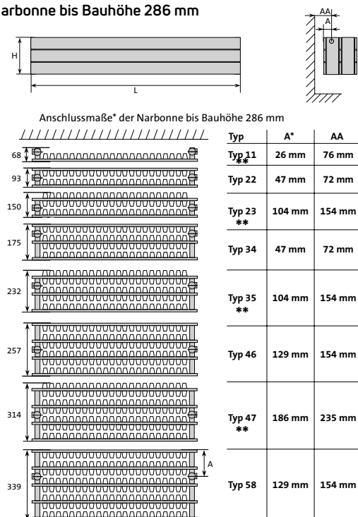
Abb. 60 Design-Heizkörper Narbonne Narbonne bis Bauhöhe 286 mm
