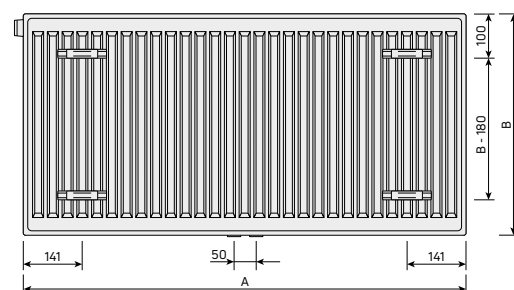
Rückansicht
