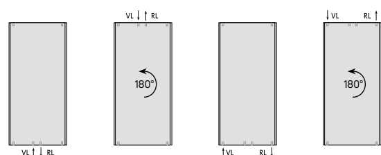
Abb. 47 Empfohlene Anschlussmöglichkeiten
