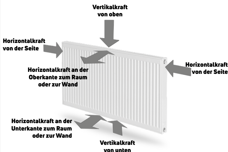
Abb. 75 Auf den Heizkörper einwirkende Kräfte
