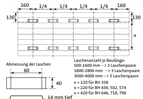
Abb. 65 Befestigung
