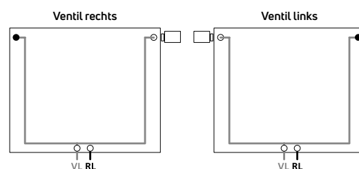
Abb. 53 Anschlusslage Ventil rechts oder Ventil links durch Ventilwechselfunktion (VL=Vorlauf; RL=Rücklauf; Vorlauf immer links!)
