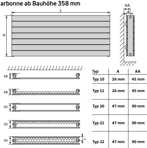
Abb. 62 Abmessungen Design-Heizkörper Narbonne ab Bauhöhe 358 mm; Abstand für Befestigungen (AA) siehe Zubehör
