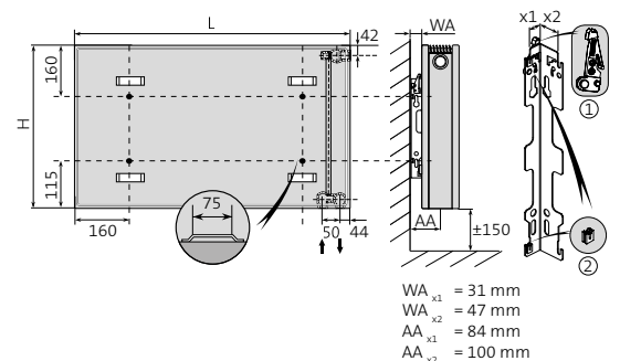
Abb. 58 Bohrmaße und Anschlüsse der Heizkörper Kos H und Faro H
