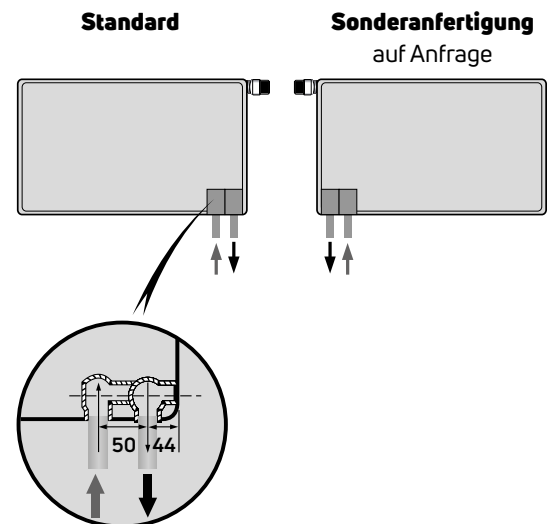
Abb. 58 Bohrmaße und Anschlüsse der Heizkörper Kos H und Faro H
