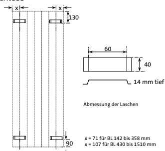
Abb. 69 Befestigung
