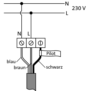
Abb. 51 Elektrischer Anschluss
