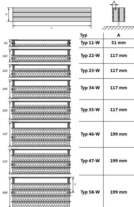
Abb. 63 Abmessungen Design-Heizkörper Narbonne mit Wärmeschutzschirm.
