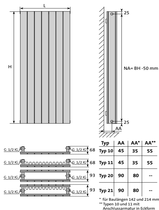
Abb. 67 Abmessungen Design-Heizkörper Narbonne V
