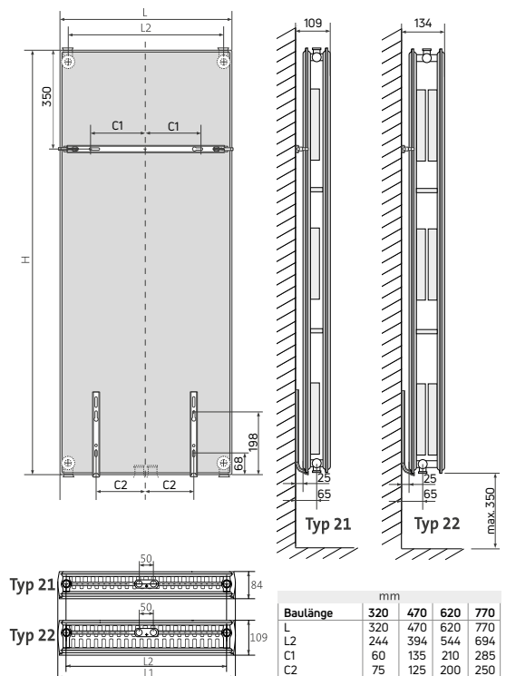
Abb. 56 Abmessungen und Befestigung Design-Heizkörper Kos V und Faro V
