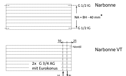
Abb. 64 Anschluss
