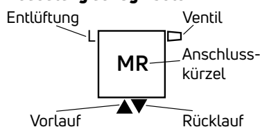
Abb. 70 Anschlussvarianten Narbonne und Narbonne VT (die jeweiligen Basispreise sind den Tabellen auf Seiten 74 bis 85 zu entnehmen; „o. VG“ = ohne integrierte Ventilgarnitur = Narbonne; „m. VG“ = mit integrierter Ventilgarnitur = Ventilausführung = Narbonne VT)
