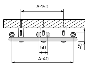
Abb. 79 Abmessungen und Montagemaße
