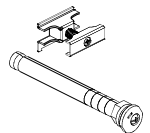
Abb. 13b Anschluss-Set mit Bohrkonsole. Das 4er-Set beinhaltet je viermal, das 6er-Set je sechsmal den unten rechts abgebildeten Umfang. Maße in mm.
