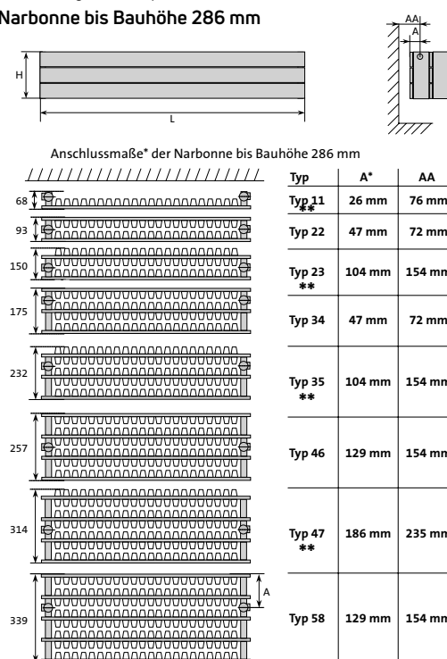
Abb. 58 Design-Heizkörper Narbonne
