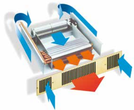
Funktionsdarstellung des Sockel-Lüfter-Konvektors OPTIMO
