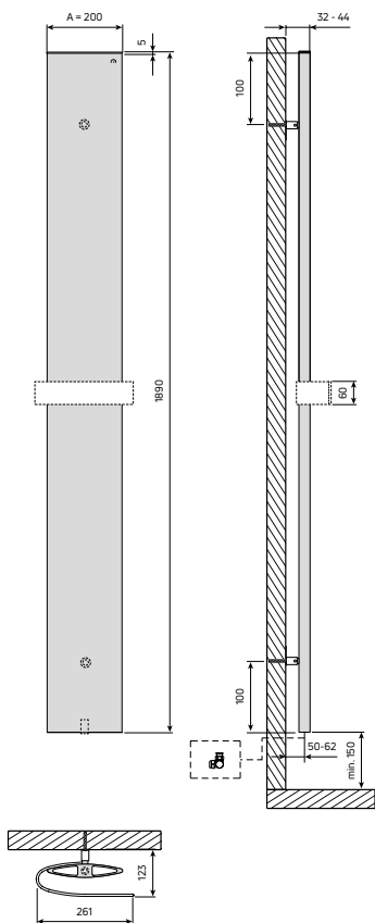
Abb. 56 Abmessungen und Montage Maße
