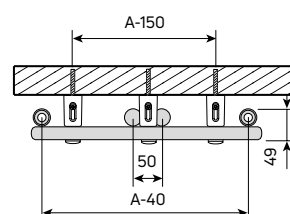
Abb. 79 Abmessungen und Montagemaße
