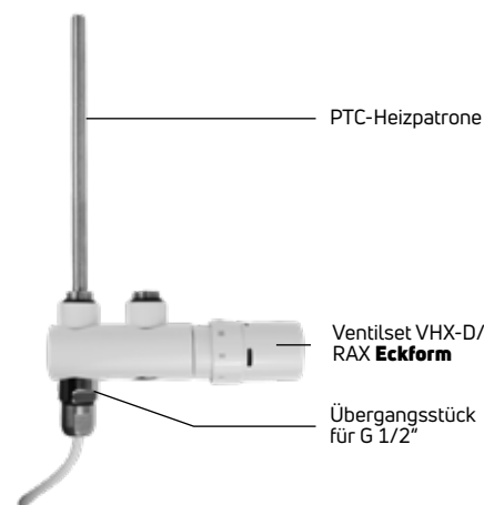
Abb. 113 Montage der PTC-Heizpatrone in Verbindung mit Ventilset VHX-D / RAX Eckform und Übergangsstück für Twist, Gate, Elato, Apolima und Evia
