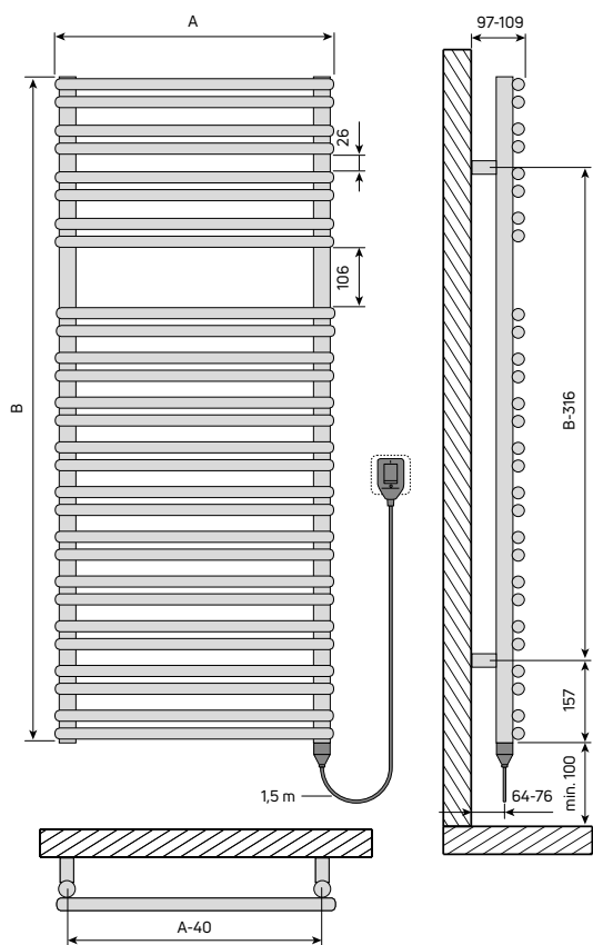
Abb. 106 Abmessungen und Montage Maße
