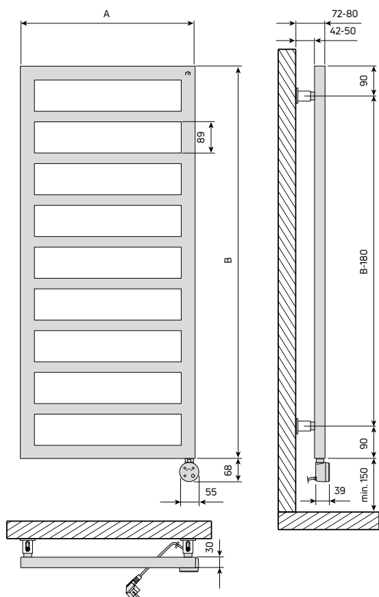
Abb. 52 Abmessungen und Montage Maße
