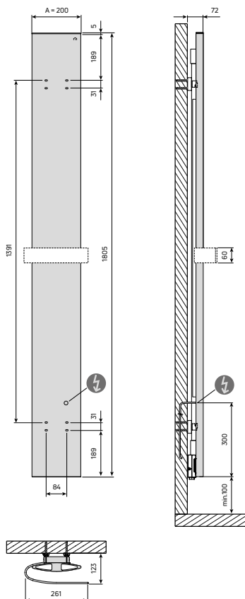
Abb. 59 Abmessungen und Montage Maße
