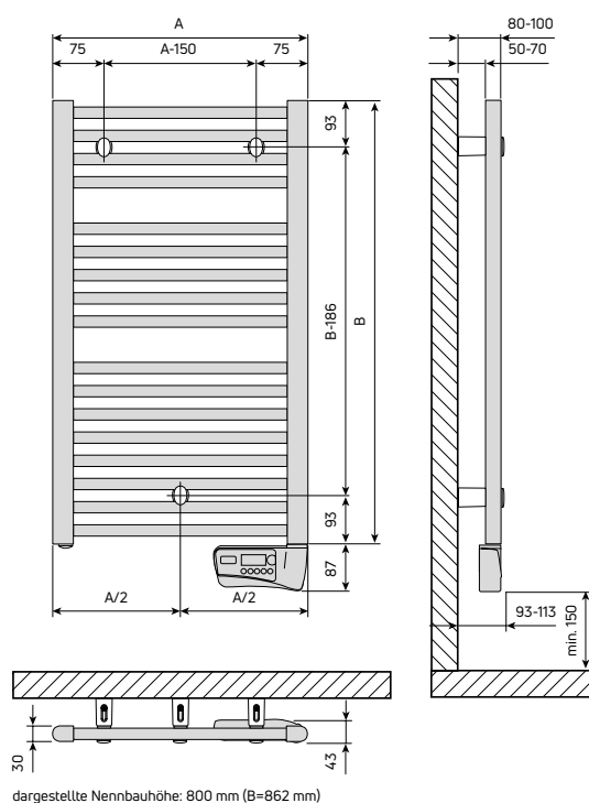
Abb. 108 Abmessungen und Montage Maße
