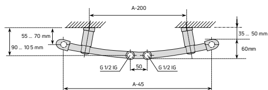
Abb. 72 Anschlussabstände Flores CM
