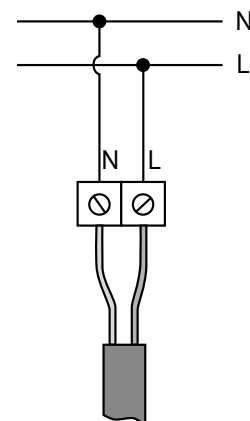
Abb. 64 Elektrischer Anschluss
