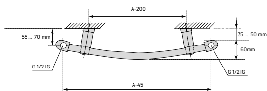
Abb. 71 Anschlussabstände Flores C
