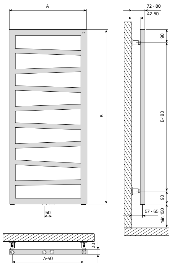
Abb. 40 Abmessungen und Montage Maße
