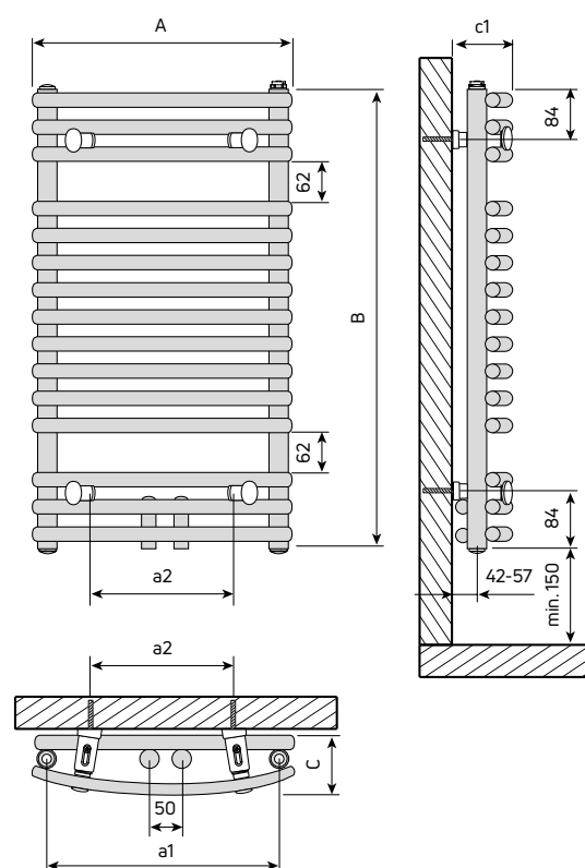
Abb. 80 Badheizkörper Santorini CM
