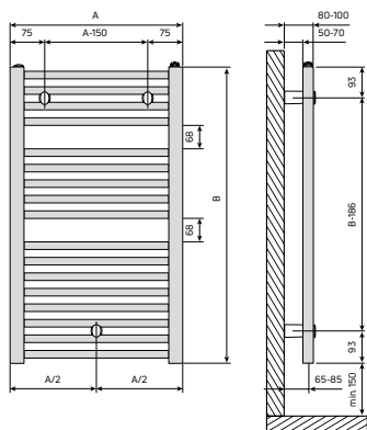
Abb. 65 Badheizkörper Flores M
