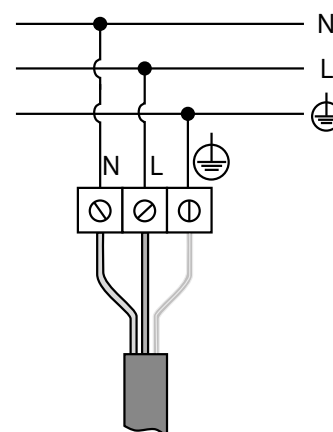
Abb. 61 Elektrischer Anschluss
