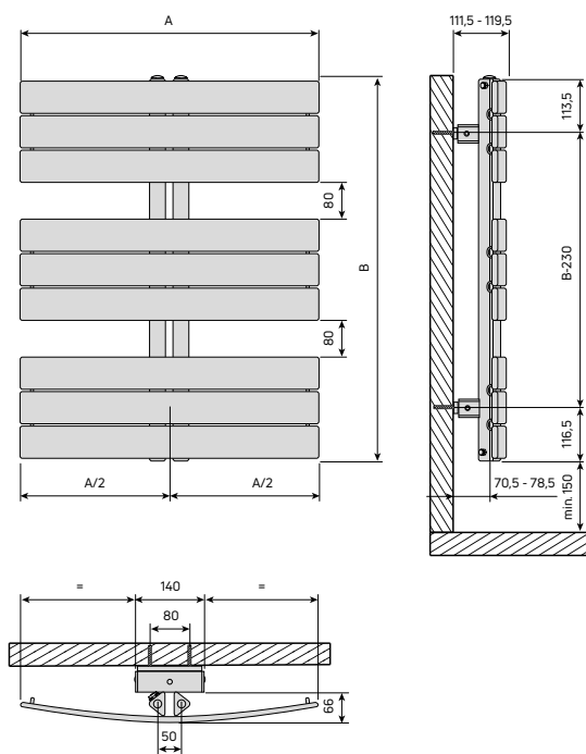
Abb. 87 Abmessungen und Montage Maße
