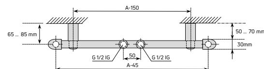
Abb. 68 Anschlussabstände Flores M
