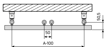
Abb. 85 Abmessungen und Montage Maße
