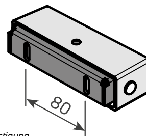
Abb. 99 Befestigung
