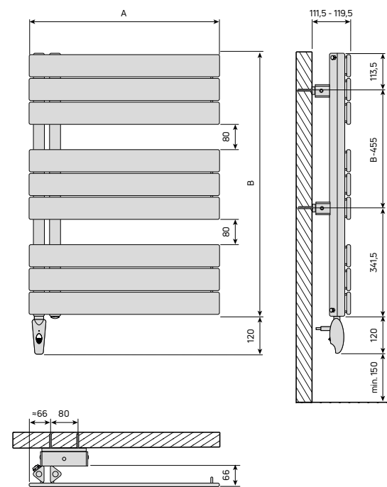
Abb. 96 Abmessungen und Montagemaße (Darstellung: Anschluss links)
