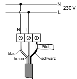
Abb. 103 Elektrischer Anschluss
