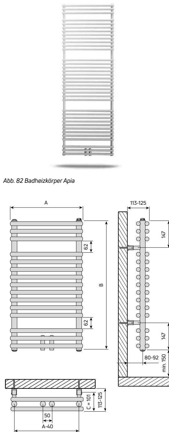
Abb. 83 Abmessungen und Montage Maße
