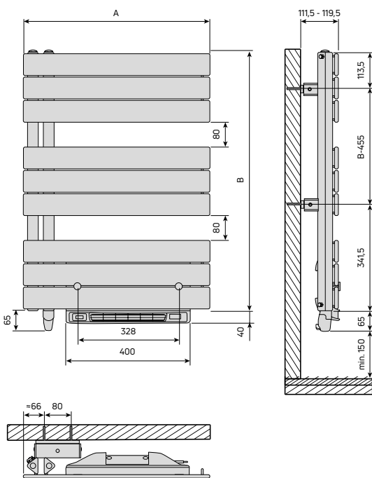
Abb. 101 Abmessungen und Montagemaße
