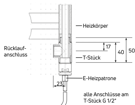
Abb. 112 Montage der PTC-Heizpatrone mit T-Stück an Heizkörpern ohne Anschluss mit 50 mm Nabenabstand (Flores und Flores C)
