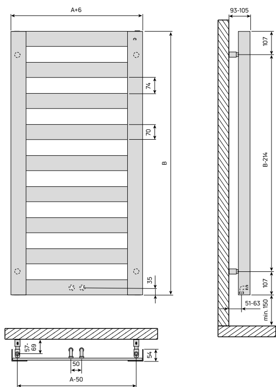
Abb. 13 Abmessungen und Montage Maße
