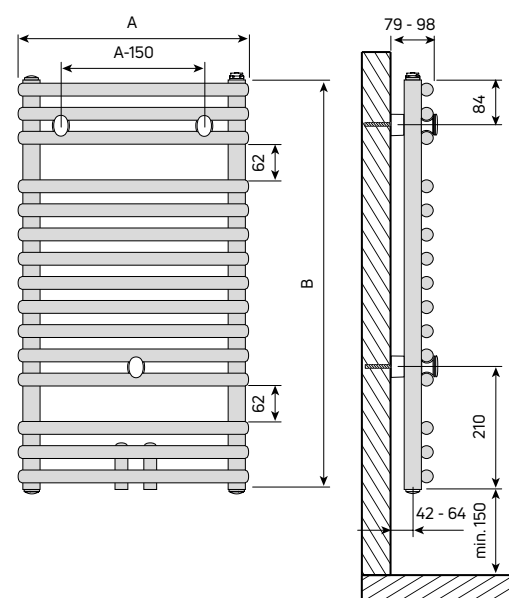
Abb. 78 Badheizkörper Santorini M
