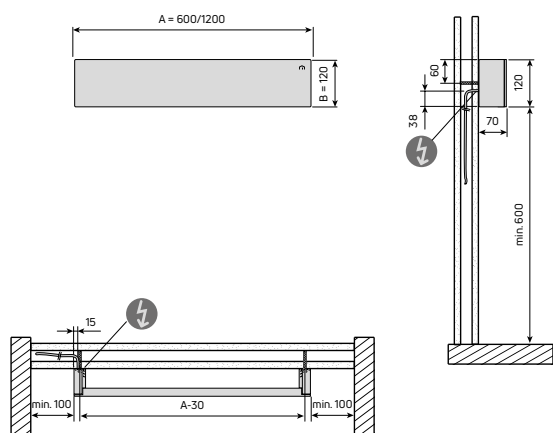
Abb. 63 Abmessungen und Montagemaße
