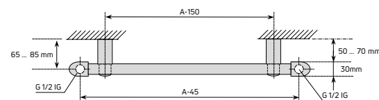
Abb. 67 Anschlussabstände Flores
