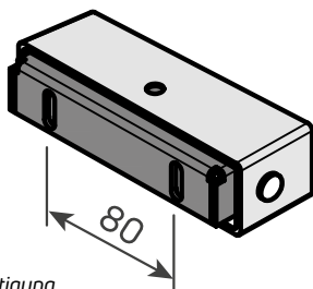
Abb. 93 Abmessungen und Montage Maße (Darstellung: Anschluss links = Standard)
