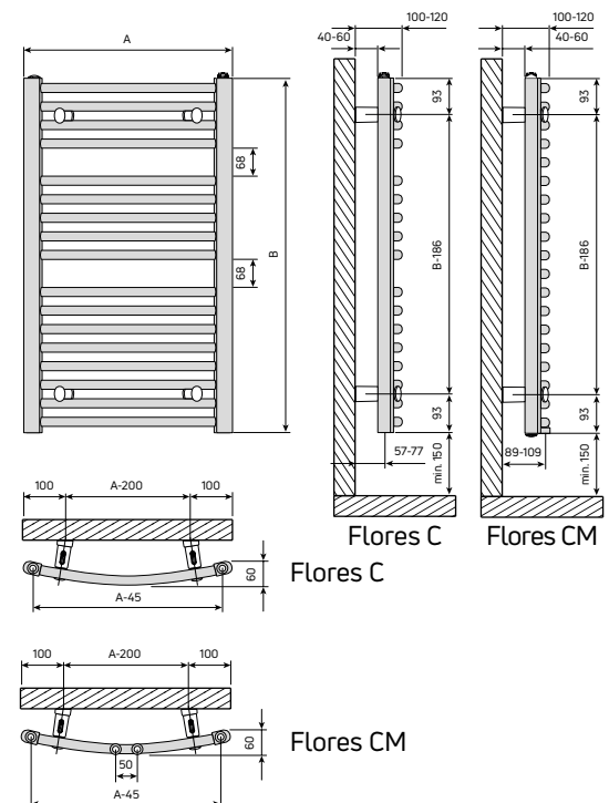
Abb. 69 Badheizkörper Flores C
