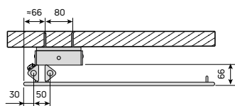
Abb. 90 Abmessungen und Montagemaße
