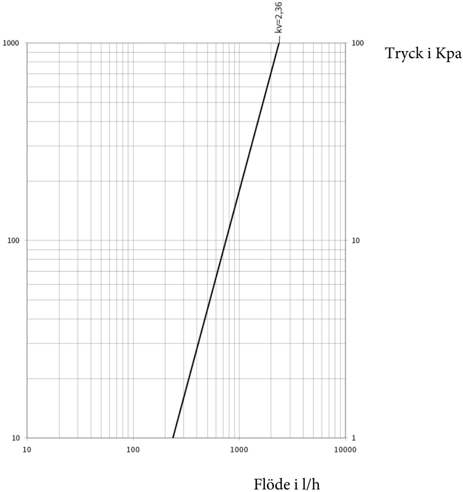
Tryckfalls diagram
