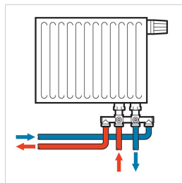
Övergång 3/4" till 1/2" AZ03TP0040013300
