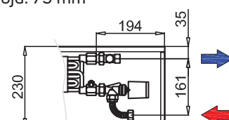
F1S-23 höjd: 75 mm
