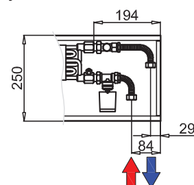
F2C-23 höjd: 110 mm
