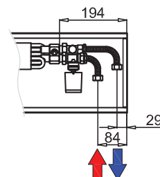
F2C-23 höjd: 110 mm
