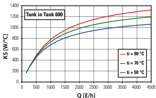
Serpentino inferiore
