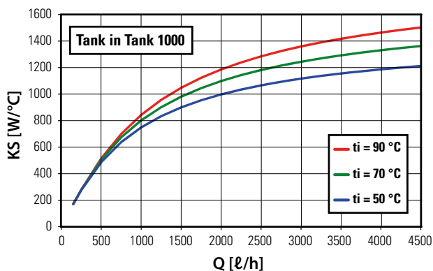
Serpentino inferiore
