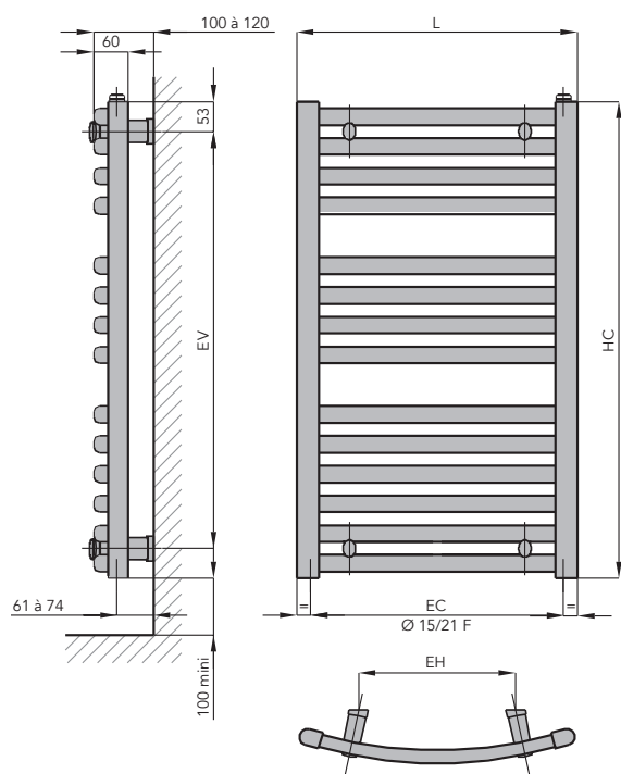
VERSION EAU CHAUDE
