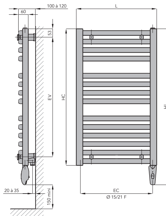
VERSIONS ELECTRIQUE ET MIXTE
