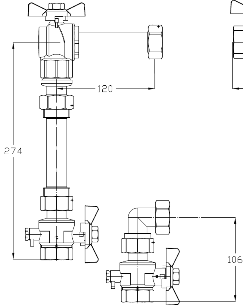
Purmo WMZ senkrecht (FBWAMWBS44F44S00)
