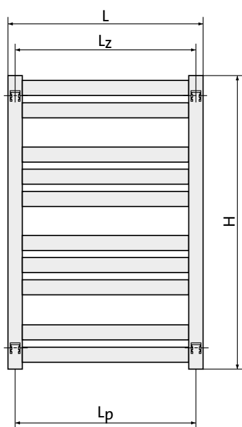
вид спереди
