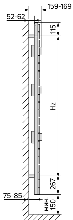
вид сбоку
