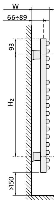
вид сбоку
