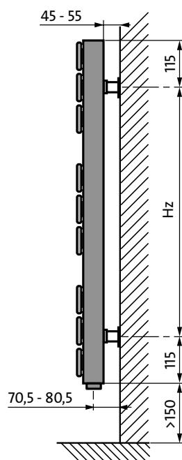
вид сбоку
