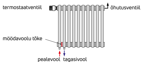
VLO ühendus (alumine vasak 1. ja 2. ribi kaudu)
