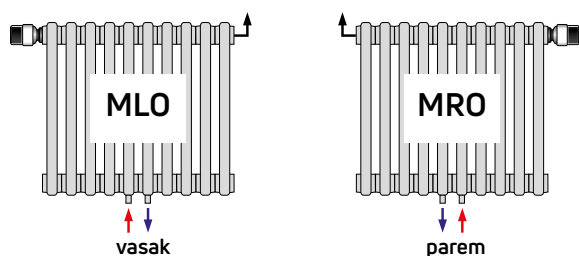
keskühendus (ainult paarisarvulise elementide arvu korral)
