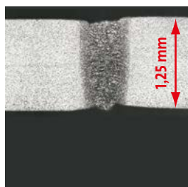
Traditsiooniliselt keevitatud ühenduste (pökk-keevitus, suurendatud vaasakul) võrdlus täiusliku Delta Laserline radiaatori ühendusega, mis on keevitatud kaasaegse lasertehnoloogiaga (suurendatud paremal).
