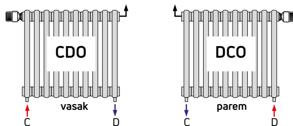
ühendus esimese ja viimase elemendi kaudu
