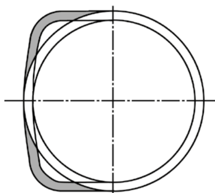
D-profilliga Delta Laserline'i radiaatori ribad, võrreldes traditsioonilise ümmarguse ribiga. Ristlõige näitab oluliselt suuremat ribi läbimõõtu. Suurenenud kogupindala (halli värviga tähistatud) tagab Delta Laserline radiaatorite suurema soojusvõimsuse.
