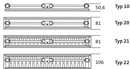
Abb. 34 Übersicht Vertical Kompaktheizkörper
