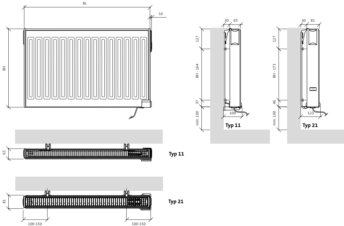
Abb. 113 Montagemaße Yali Digital
