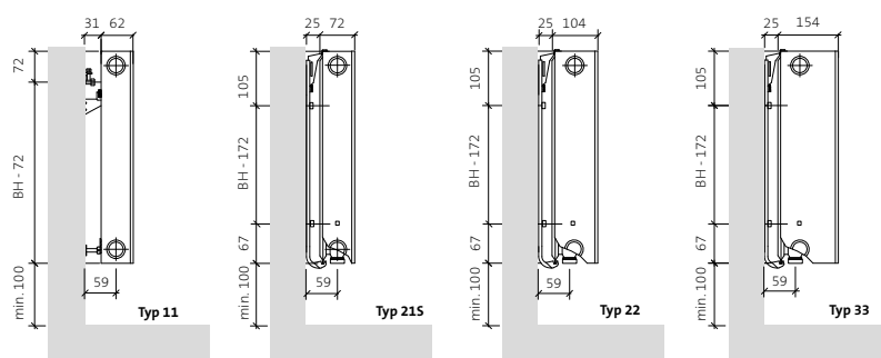
Abb. 59 Montagemasse und Anschlusslage Plan Ventil Compact M
