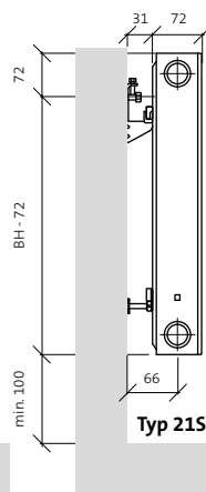
Montagemaße für Plan Compact mit Befestigungslaschen
