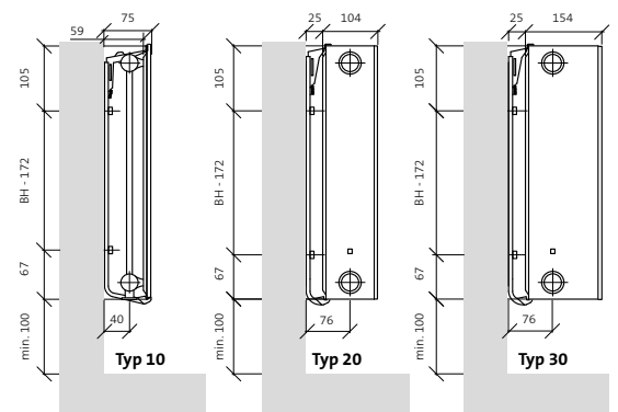
Abb. 83 Montage Maße für Plan Ventil Compact Hygiene
