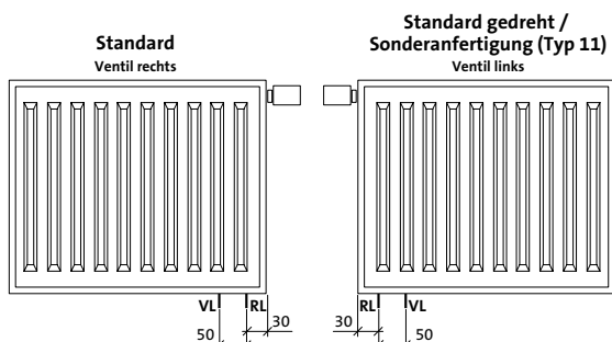
Abb. 18 Anschlusslage Ventil rechts und Ventil links
