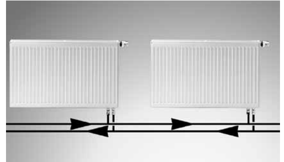
Abb. 88 2-Rohr-System
