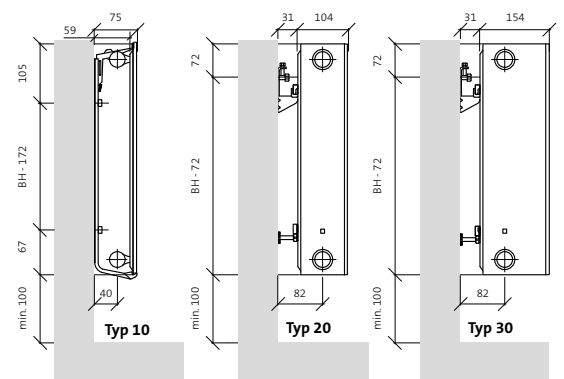
Abb. 82 Montage Maße für Plan Compact Hygiene
