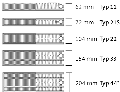
Abb. 72 Übersicht Ramo Ventil Compact
