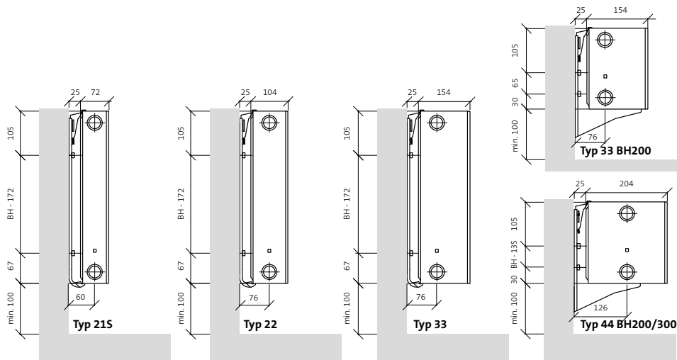
Abb. 74 Montagemaße für Ramo Ventil Compact Typen 215, 22, 33 und 44
