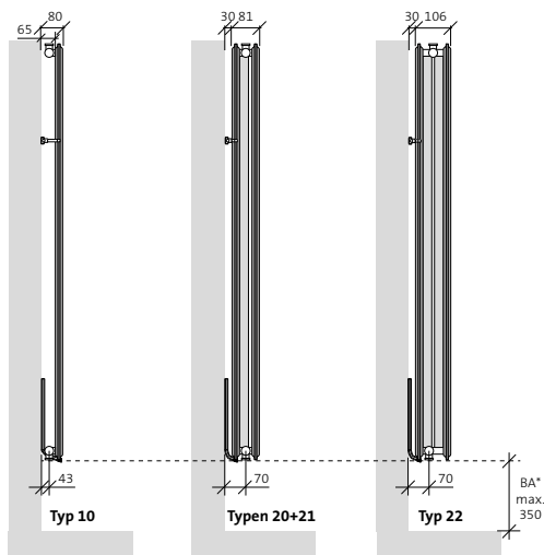
Abb. 36 Montage- und Anschlussmaße Vertical Kompaktheizkörper
