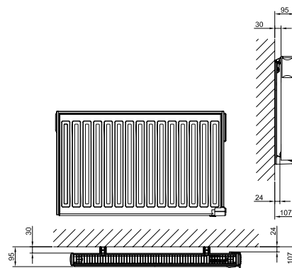
• Enkel radiator
