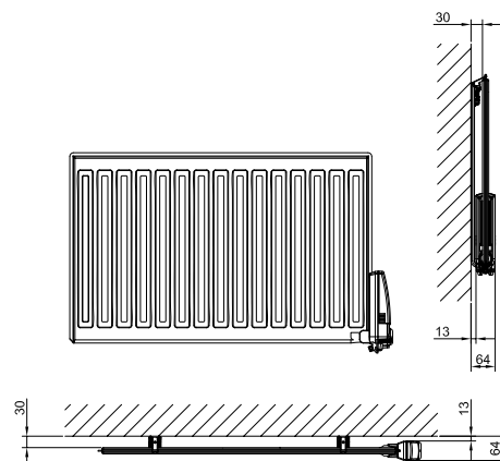
• Enkel radiator
