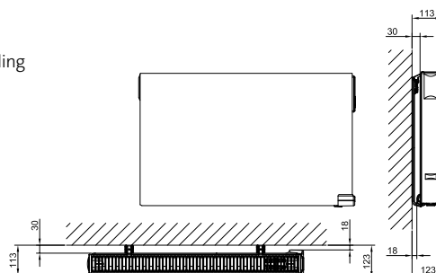
• Doble radiator
