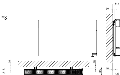
• Doble radiator
