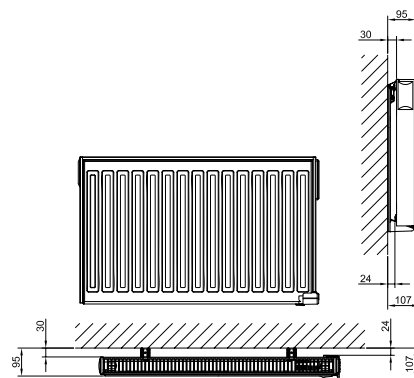
• Enkel radiator
