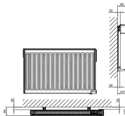
• Enkel radiator
