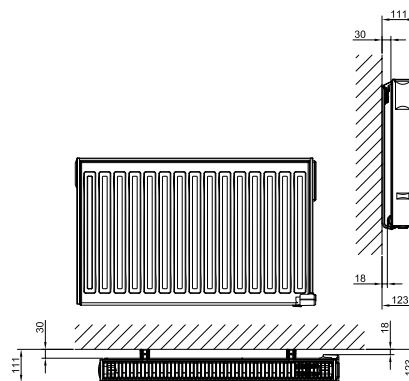
• Doble radiator
