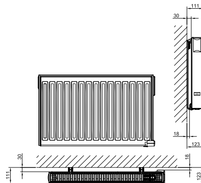
• Doble radiator
