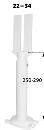
Purmo Kon forlænget gulvkonsol. Pakkes parvis. Incl. luftskrue og prop.
