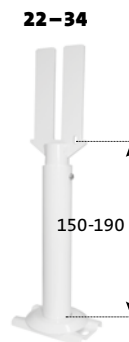
Purmo Kon H150-190 gulvkonsol. Pakkes parvis. Incl. luftskrue og prop.
