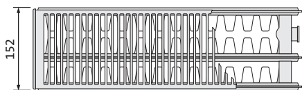
PURMO C 33
