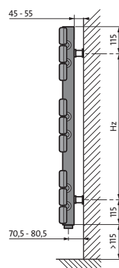
oldalnézet
