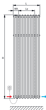
előlnézet
