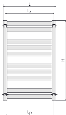
előlnézet
