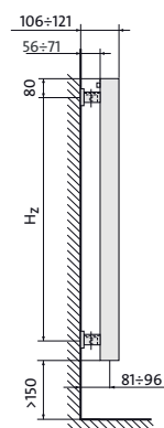
oldalnézet
