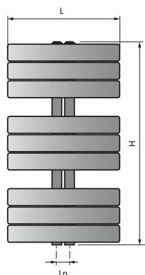
előlnézet
