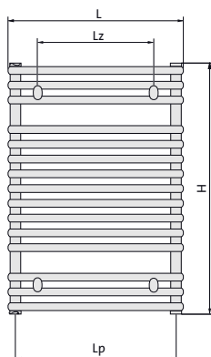
előlnézet
