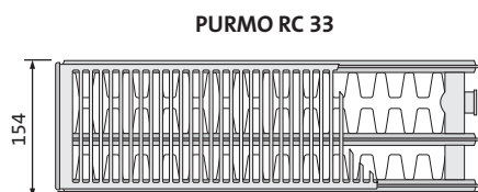
PURMO RC 33
