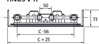
TINOS V 11
