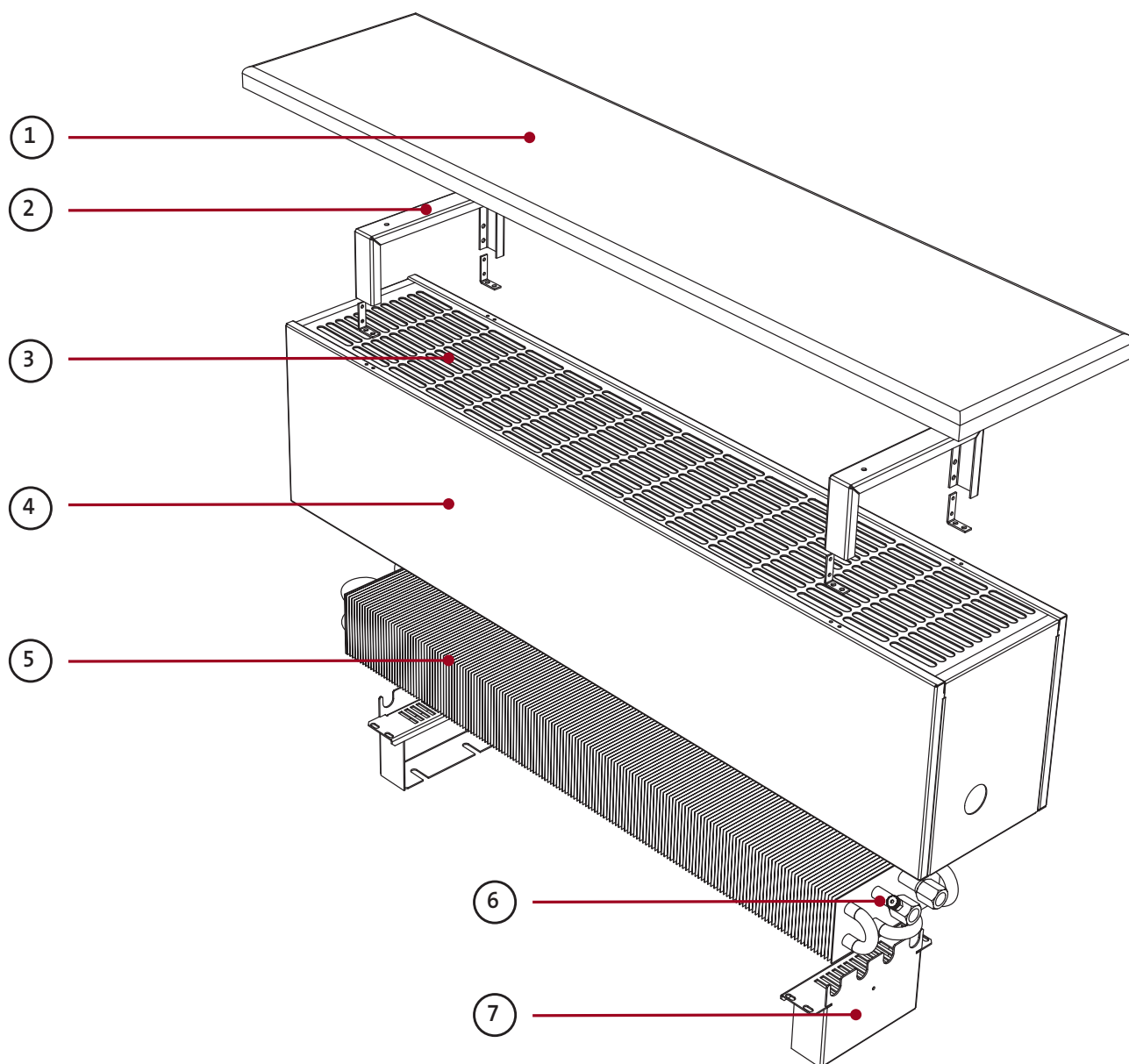
Устройство конвектора Aura Bench
