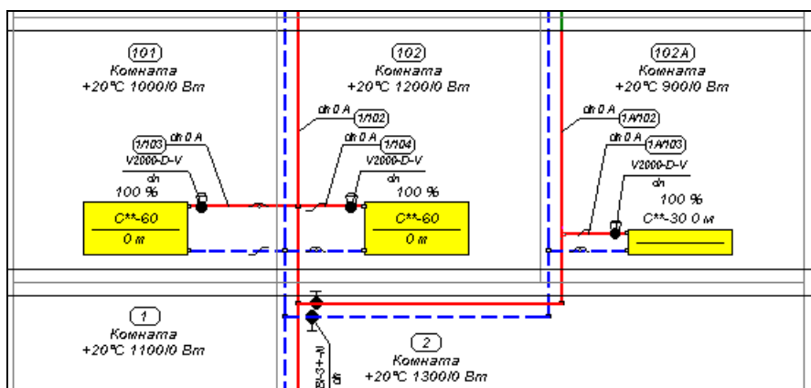
Рис. 9.19. Подсоединение стояка 1А со стояком ном. 1
