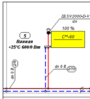
Рис. 9.17. Фрагмент рисунка с отопительным прибором, подключенным при помощи соединительного элемента RTD-K
