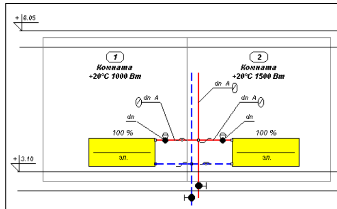
Рис. 5.28. Фрагмент схемы с нарисованными этикетками трубопроводов и арматуры
