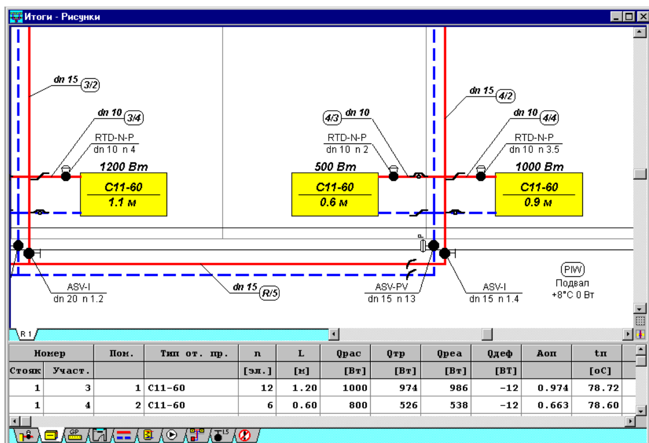
Рис. 9.14. Фрагмент схемы с итогами расчетов
