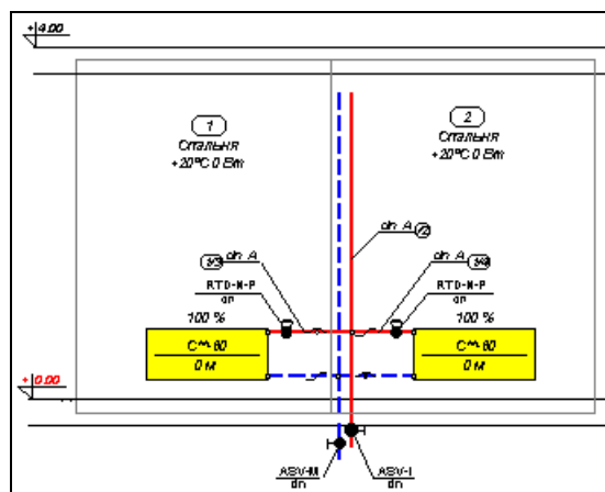
Рис. 9.7. Вставленный фрагмент этажестояка с заполненными данными
