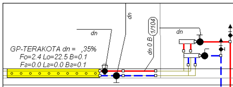
Рис. 5.54. Расположение регулирующих вентилей рядом с подпольным отопительным прибором.
