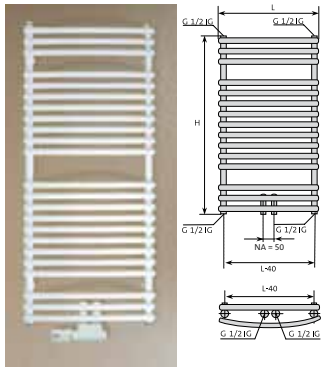
Santorini CM mit gebogenen aufgesetzten Rundrohren
