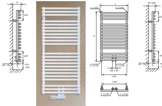
Santorini M mit geraden aufgesetzten Rundrohren
