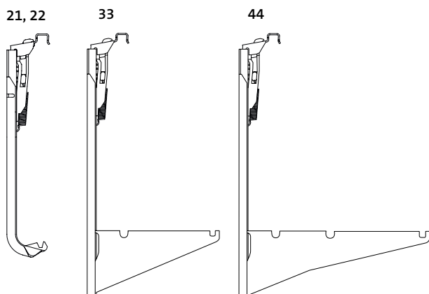
PURMO Monclac-veggkonsoll (h. 200). Typene 21-22 bestilles parvis inkl. blindplugg og lufteskruer. Typene 33 og 44 stykkevis. Lufteskruer og blindplugg inngår ikke med type 33 og 44.
