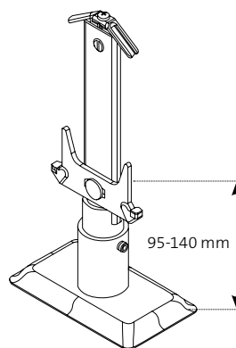
PURMO Monclac-gulvkonsoll (h. 200). Pakket stykkevis. Lufteskruer og blindplugg inngår ikke.
