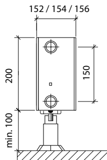
CV 33 típus FCV 33 típus RCV 33 típus FFCV 33 típus RRCV 33 típus
