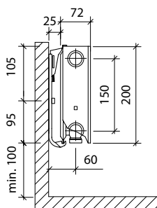
FCV 21 s típus RCV 21 s típus
