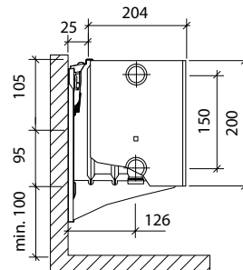
FCV 44 típus RCV 44 típus
