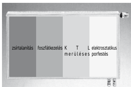
A fűtőtestek felület-előkészítése
