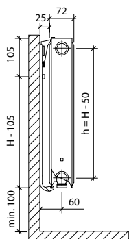
FCV 21 s típus
