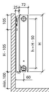
RCV 21 s típus
