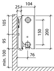
FCV 22 típus RCV 22 típus
