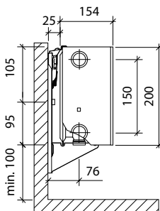
FCV 33 típus RCV 33 típus
