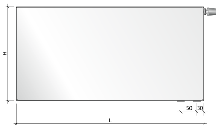
Szerelési távolságok [mm]:
