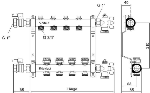
Heizkreisverteiler Standard
