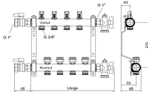
Heizkreisverteiler mit Durchflußmengenmesser
