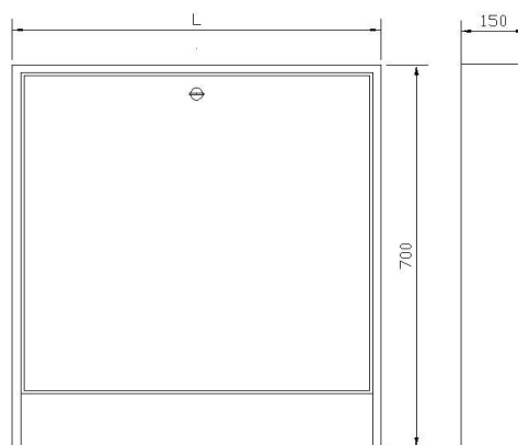
Heizkreisverteilerschrank Aufputz
