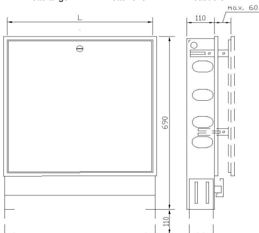
Heizkreisverteilerschrank Unterputz
