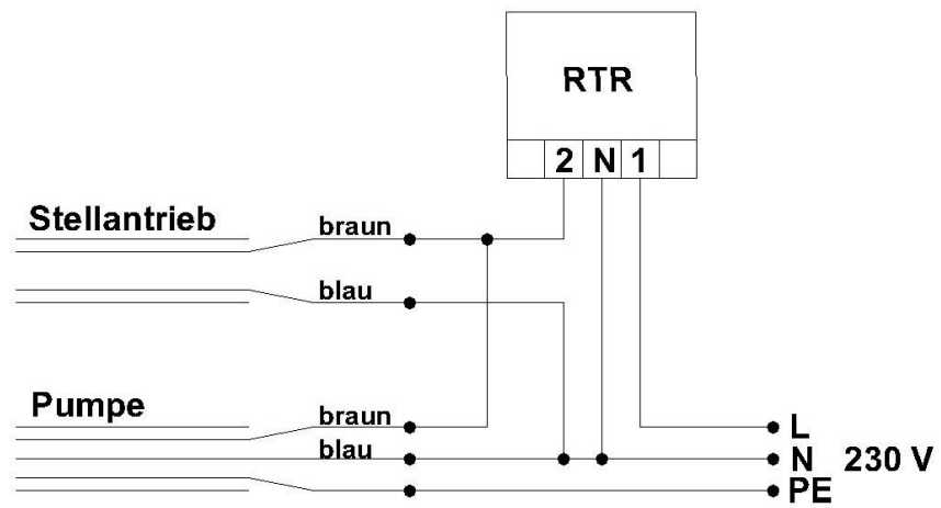
Pumpe durch Raumthermostat RTR geschaltet
